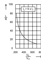
DC-Anwendung DC-Application
