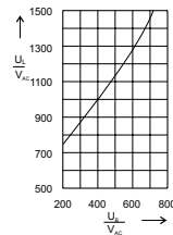
Schaltspannungsdiagramm Arc Voltage-Diagram
