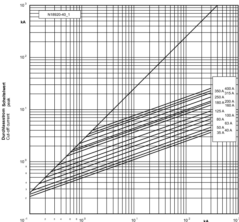
unbeeinflusster Kurzschlussstrom Prospective short-circuit-current (Sym. r.m.s.)
